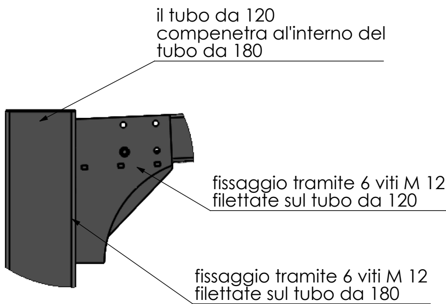
DETTAGLIO D SCALA 1 : 10
