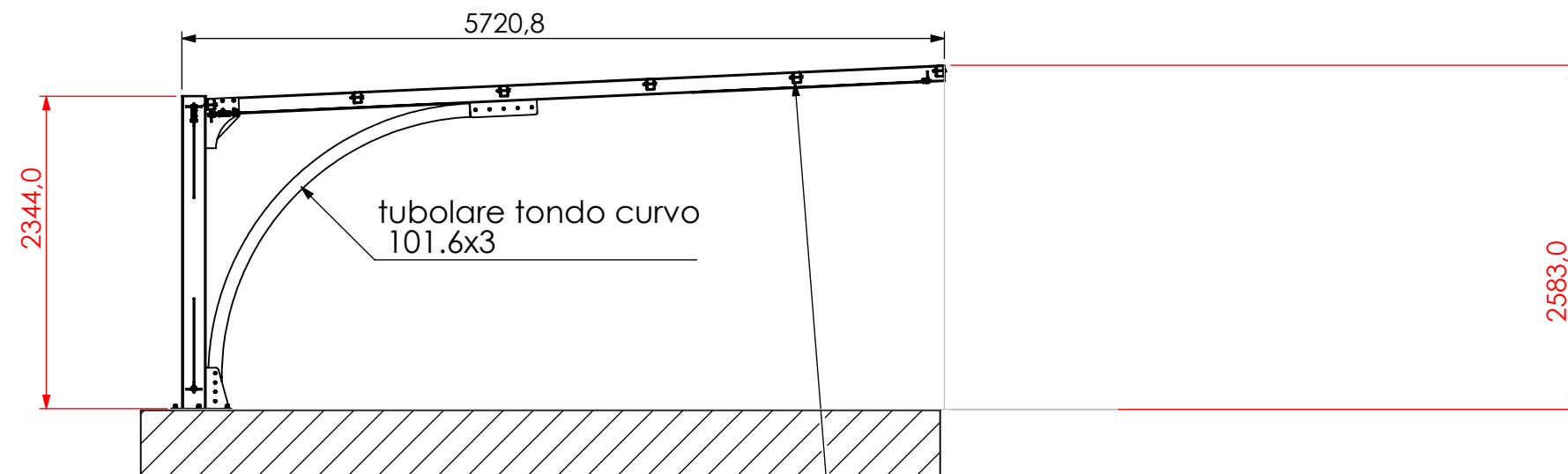
SEZIONE A-A
