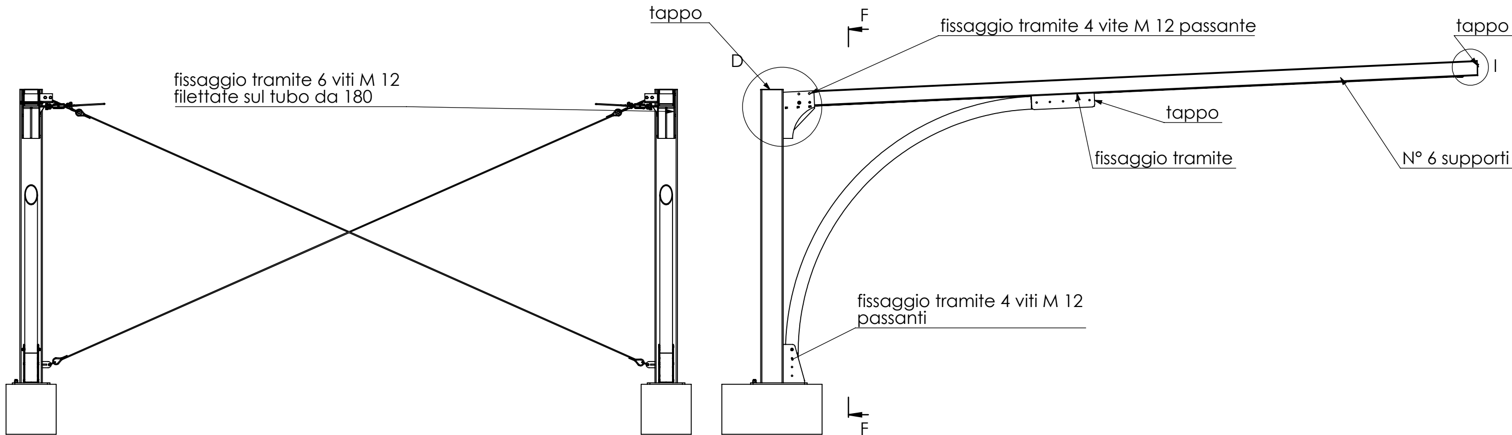
SEZIONE F-F
